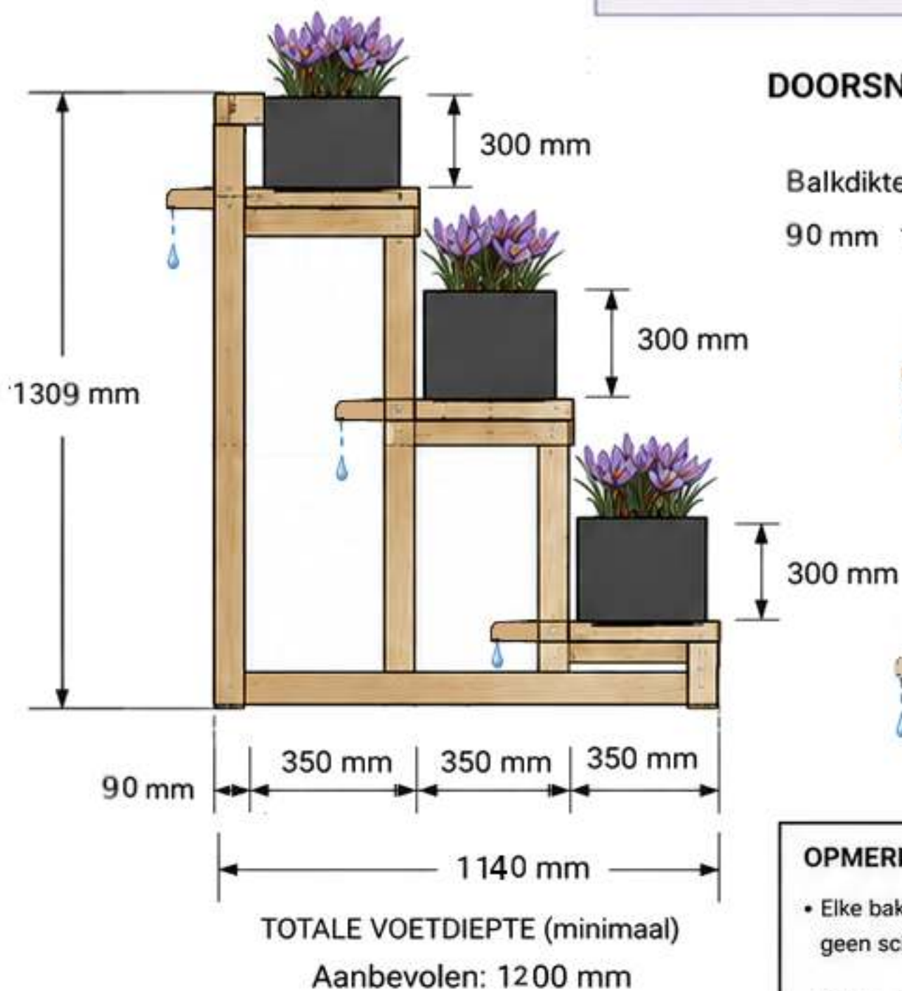
ZIJAAANZICHT
