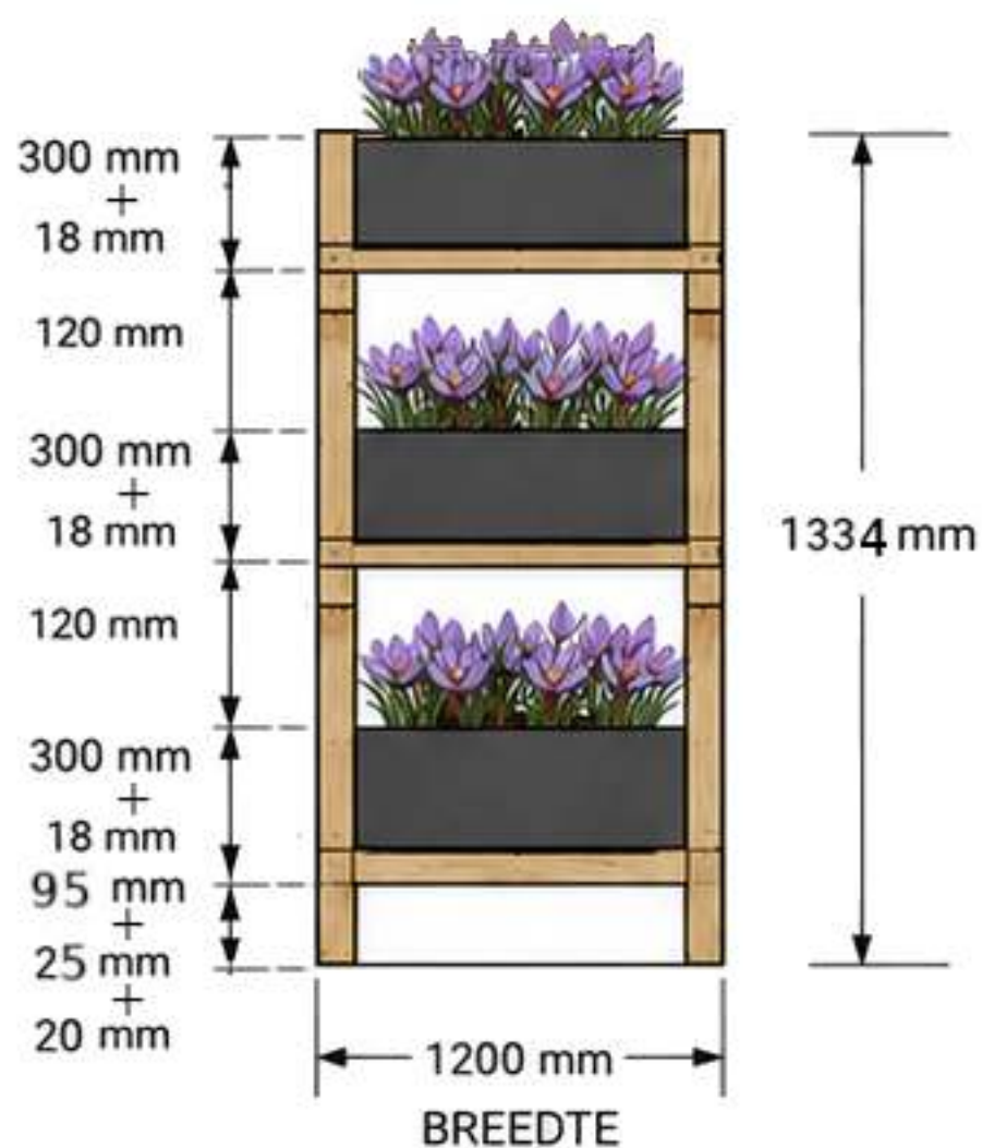
VOORAANZICHT
