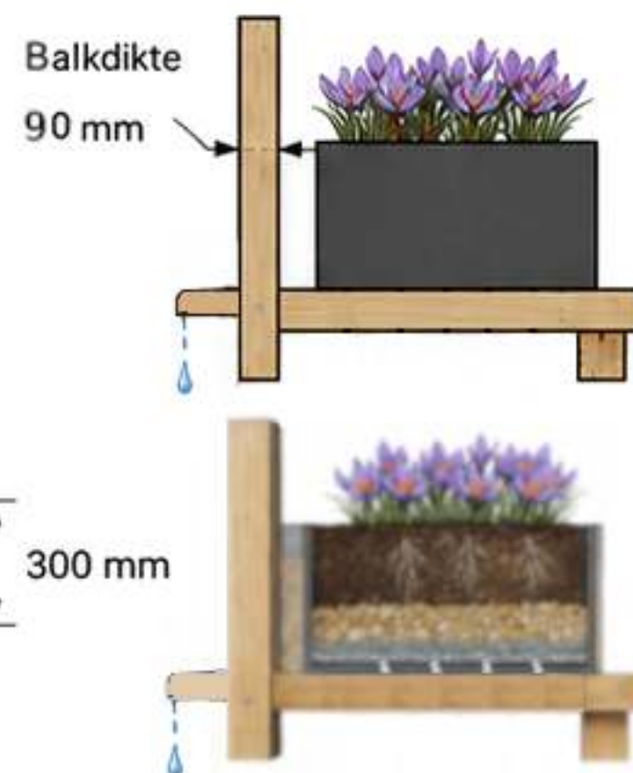
DOORSNEDE / DETAILS
